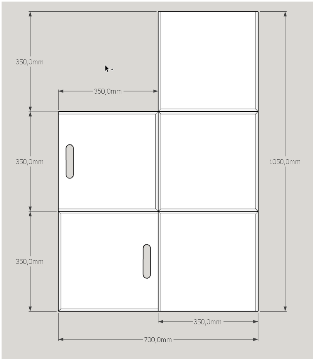
Die Bauteile der Innenkiste für einen Plattenzuschnitt.
